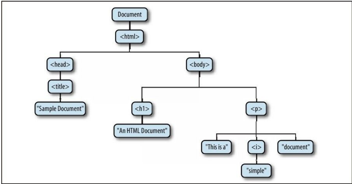
图 15-1 HTML文档的树状表示
