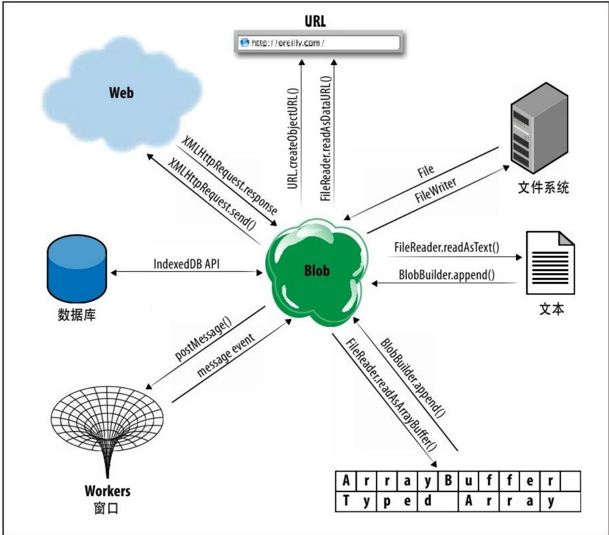
图 22-2 Blob以及使用Blob的API
