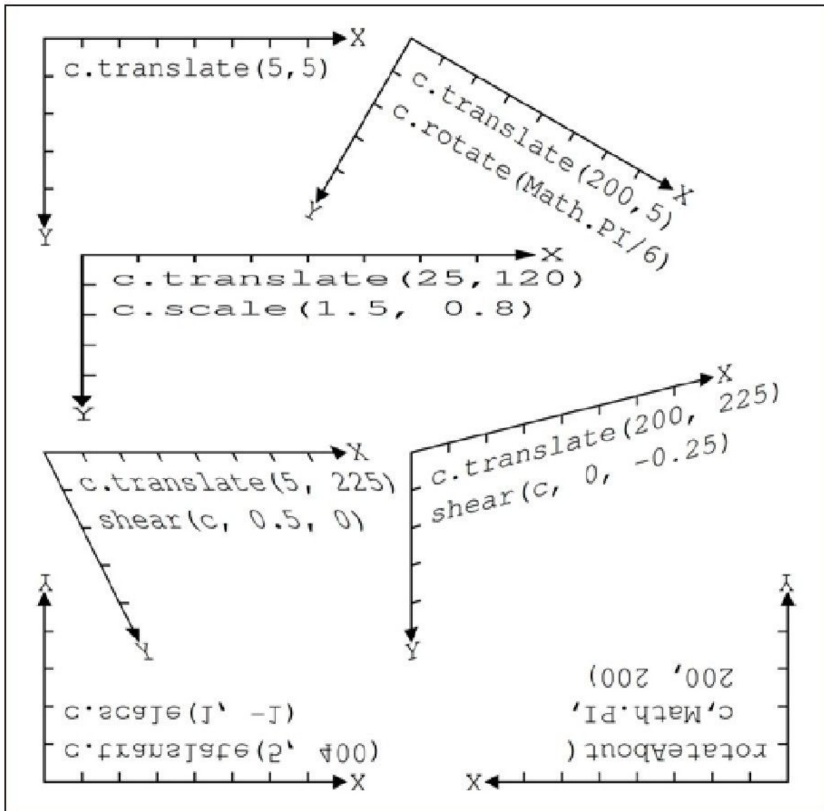
图 21-7 坐标系变换
