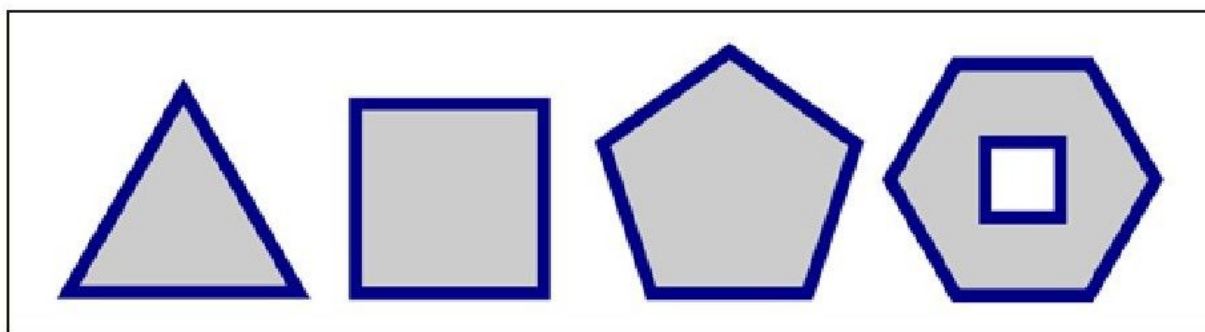
图 21-6 规则多边形
