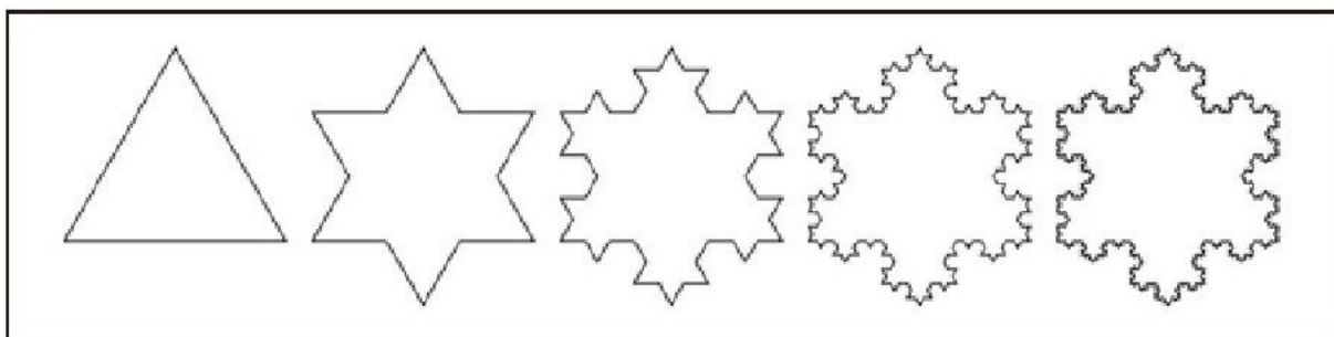
图 21-8 科赫雪花
