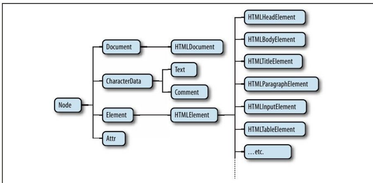
图 15-2 文档节点的部分层次结构
