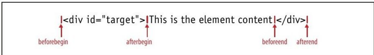
图 15-3 insertAdjacentHTML()的插入点
